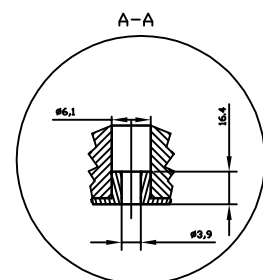
Otwór do mocowania gniazda
