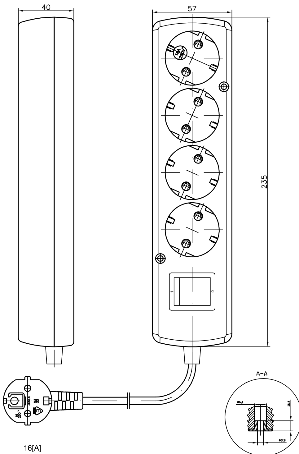
Otwór do mocowania gniazda
