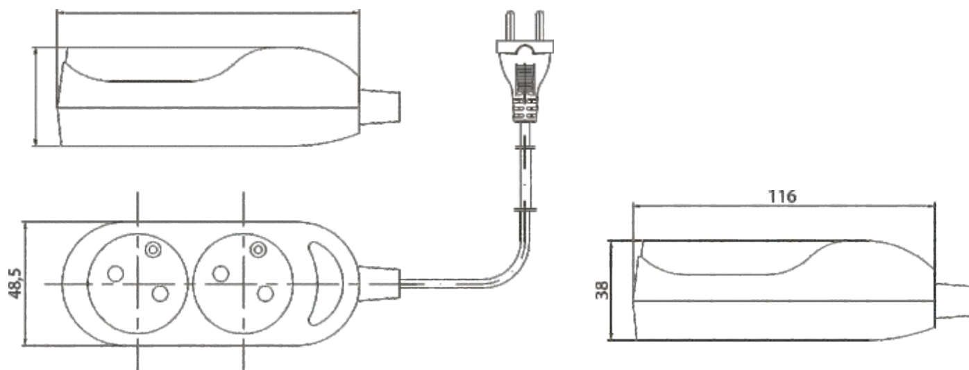
Przedłużacz z dwukrotnym gniazdem
